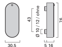
Dornrosette mit Dornloch und Verdeck, senkrecht DRS Rose with aperture and swing cover (vertical) DRS
