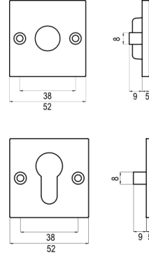
Quadratrossetten KR
