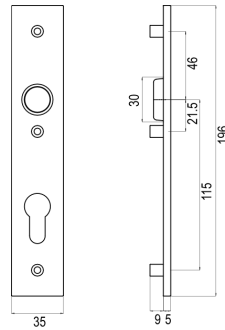
Kurzschild KK3
