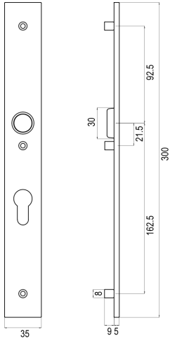
Langschild KL2
